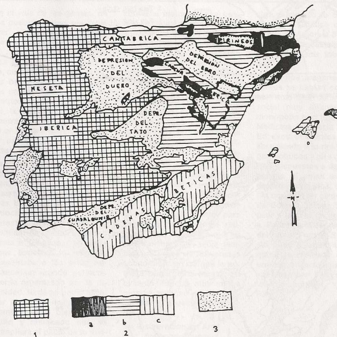
Fig. 3 — Situación de la provincia de Teruel en las grandes unidades de la Península Ibérica. 1: Hercínico de la Meseta 2: Cadenas alpinas. a: Paleozoico, b: Mesozoico, c: Paleozoico y Mesozoico de las Béticas. 3: Depresiones terciarias.
