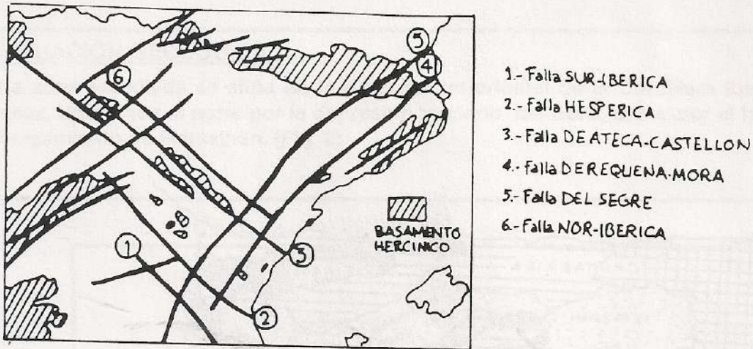
Fig. 4: Esquema estructural y principales accidentes tectónicos hercínicos del área Ibérica (según SIMON, 1986).
